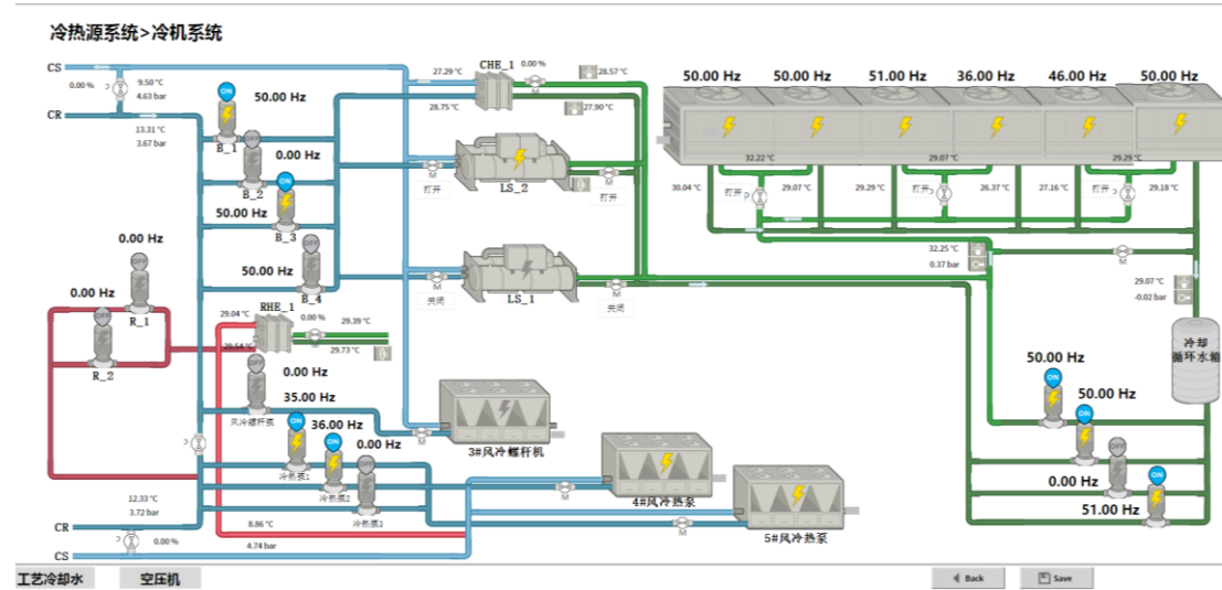
冷热源控制系统
