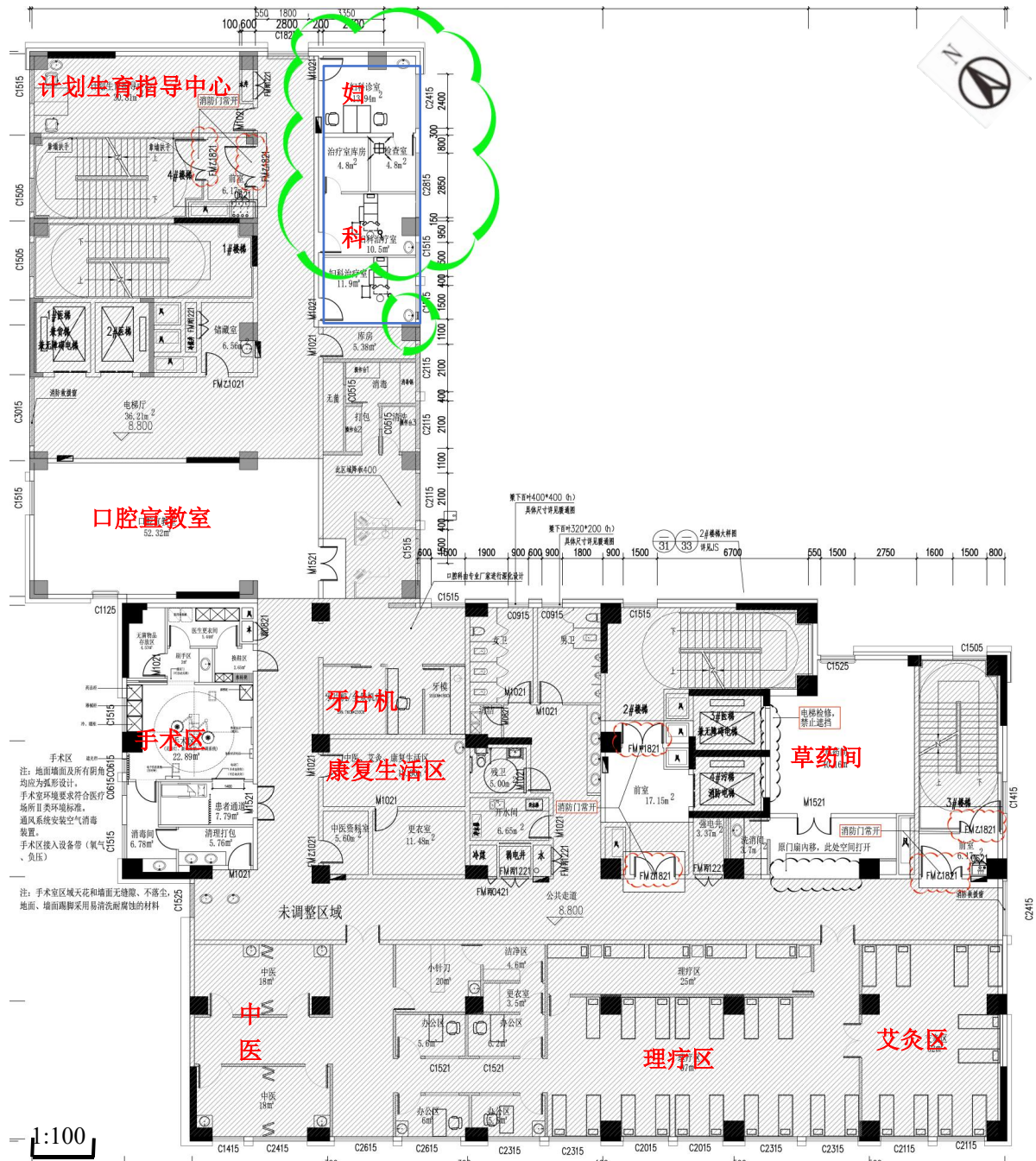
附图 6-4 三层平面布置图
