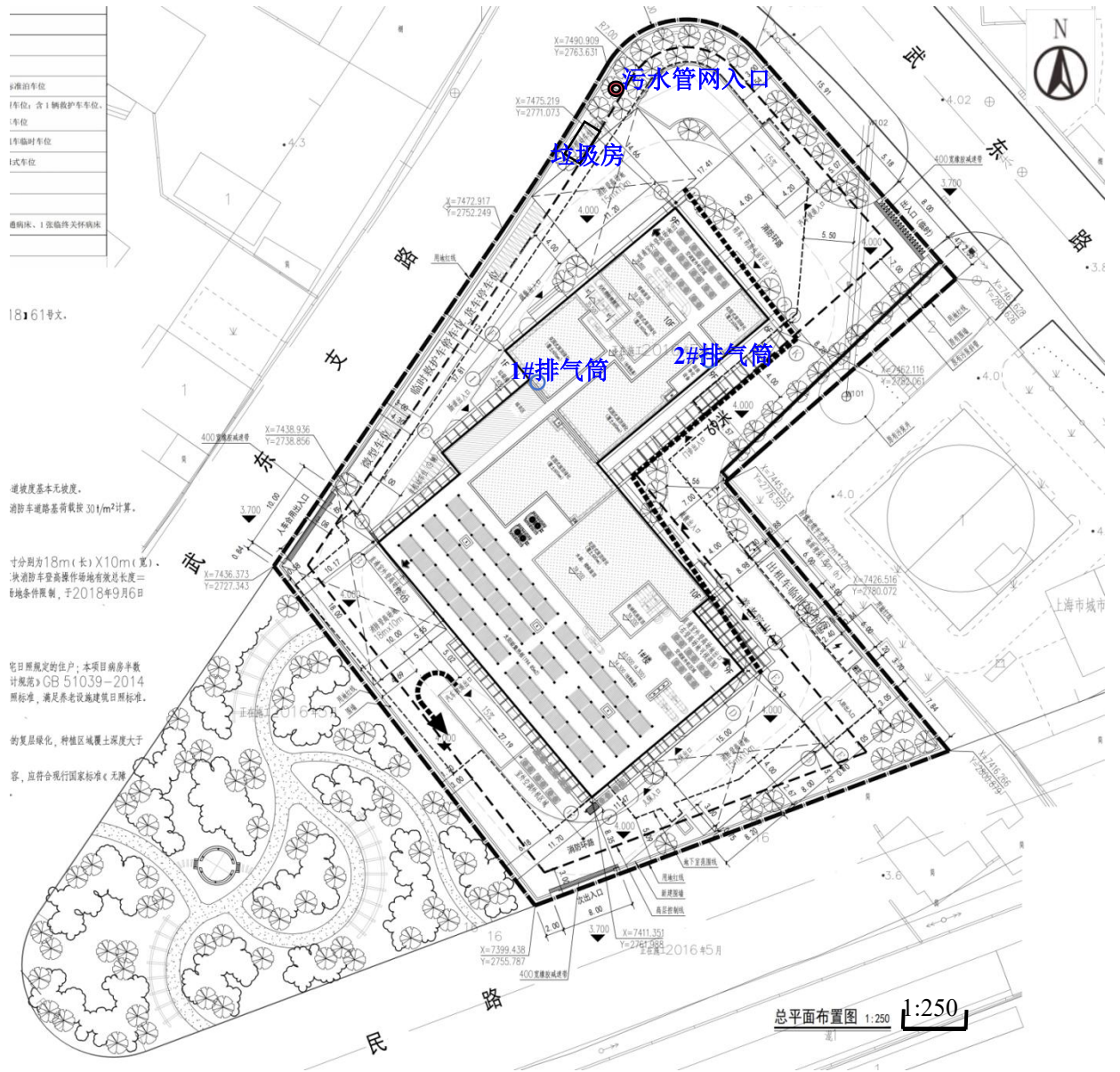
附图5 项目总平面布置图
