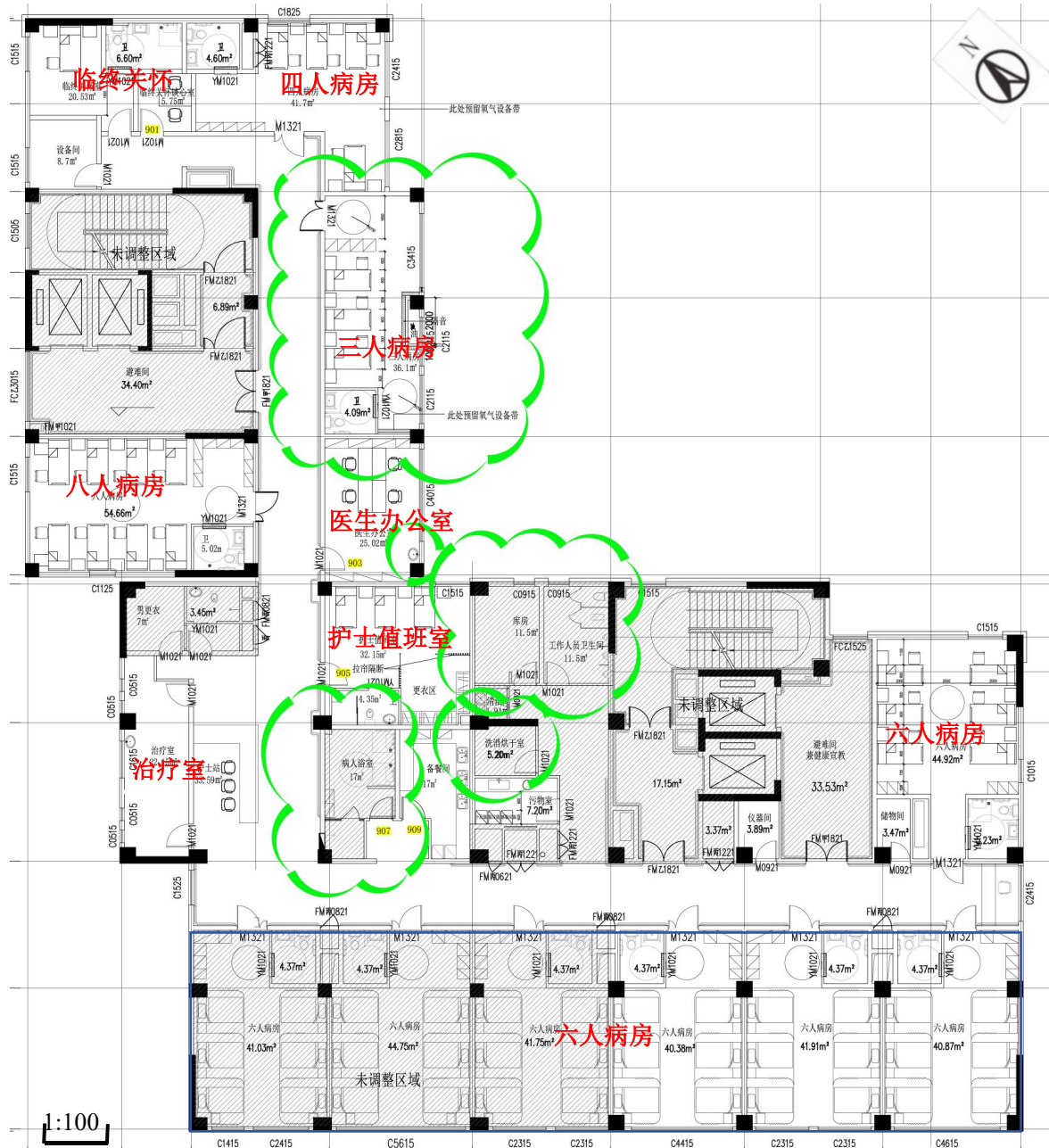
附图 6-10 九层平面布置图
