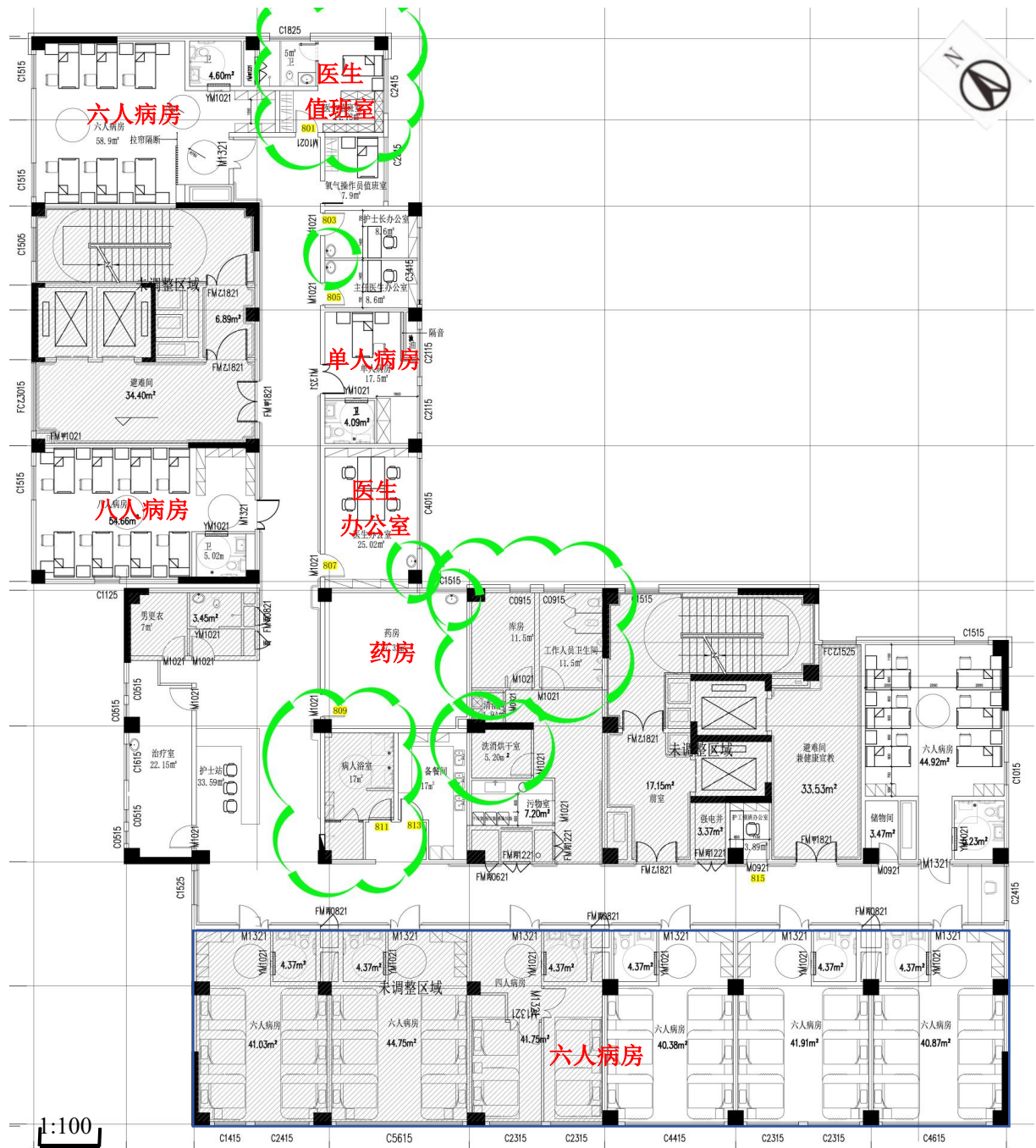
附图 6-9 八层平面布置图
